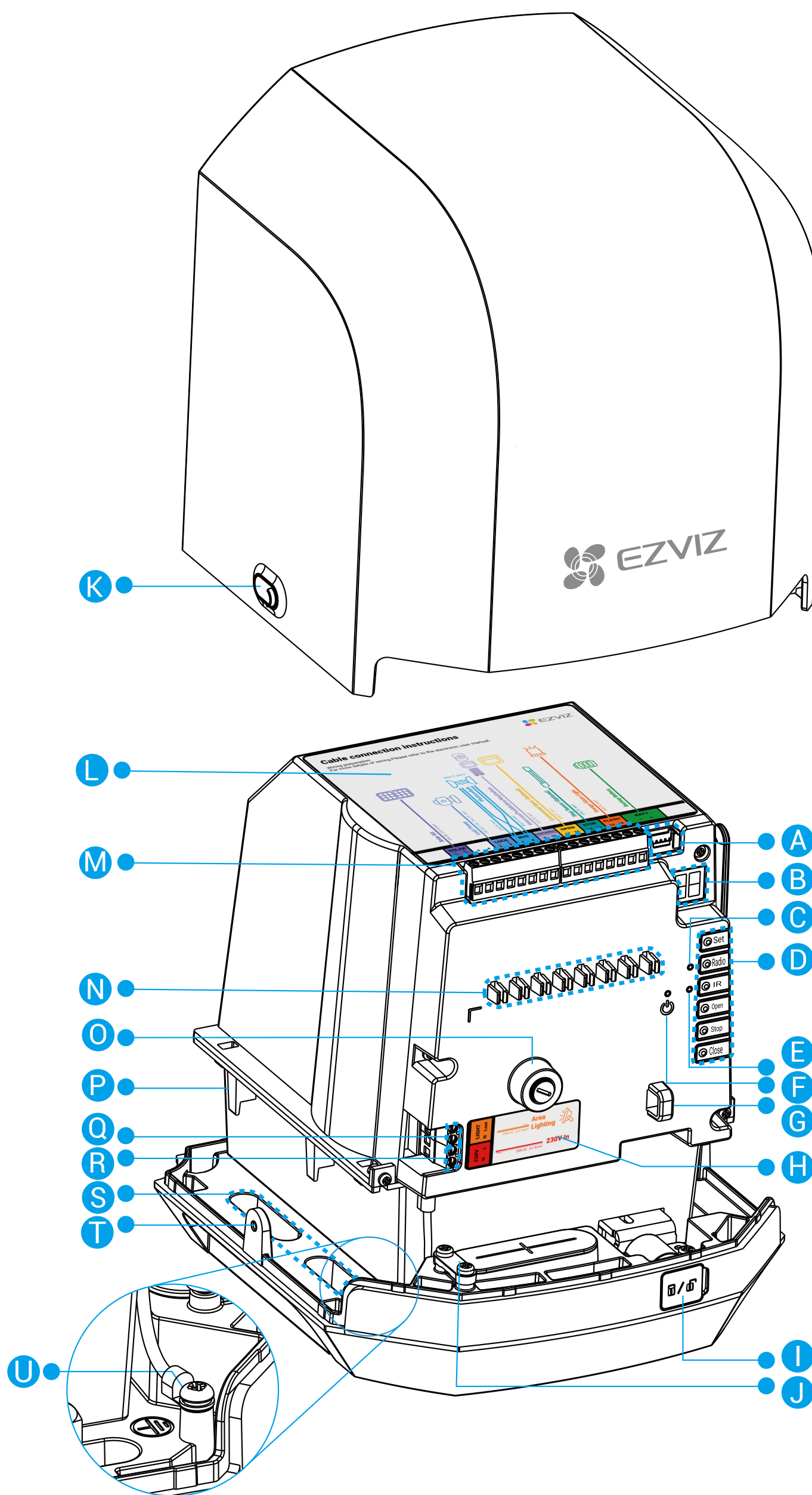
Prednji prikaz
