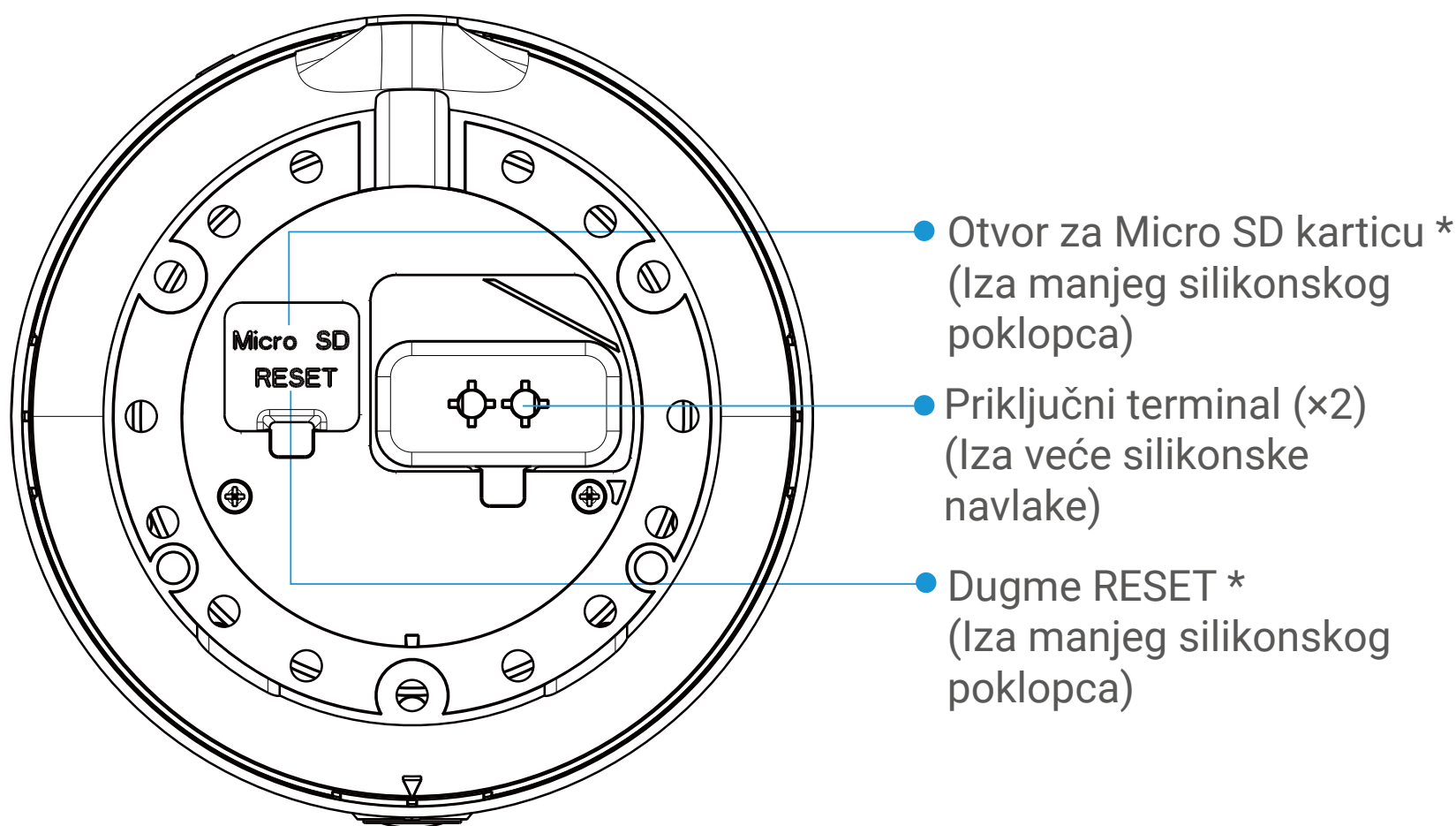
Donji pogled
